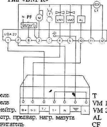
ЭЛЕКТРОСХЕМА ВНУТРЕННЕГО СОЕДИНЕНИЯ
