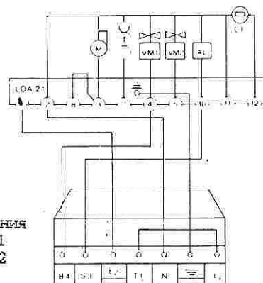
ЭЛЕКТРОСХЕМА ВНУТРЕННЕГО СОЕДИНЕНИЯ
